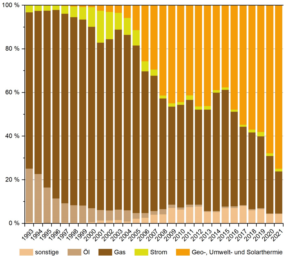
Anteile der Heizenergien im Wohnungsneubau in Sachsen-Anhalt seit 1993
